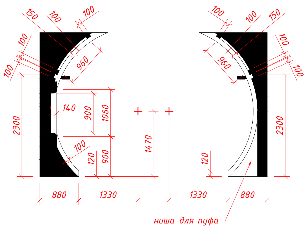
РАЗРЕЗ А-А
