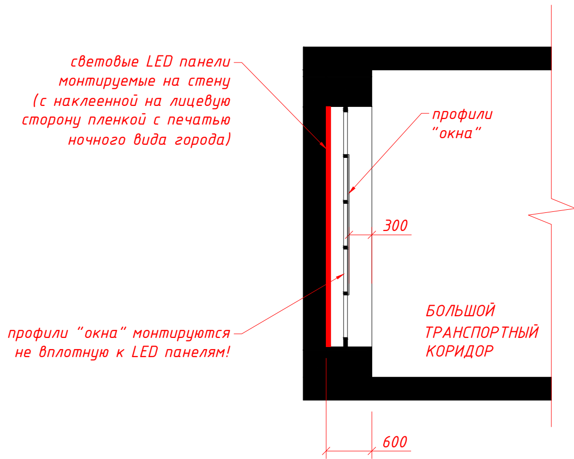
РАЗРЕЗ ПО "ОКНУ"
